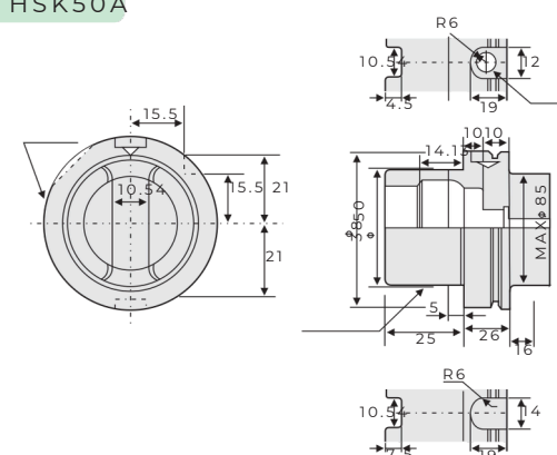
HSK50A
