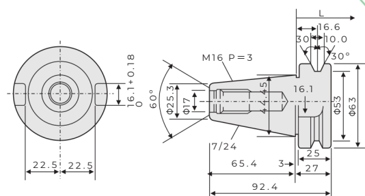
Bt40
