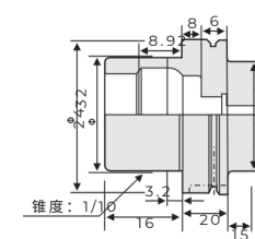
HSK32E
