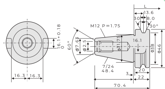
Bt30
