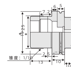
HSK25E
