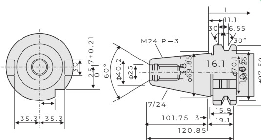
Sk50
