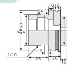
HSK50E
